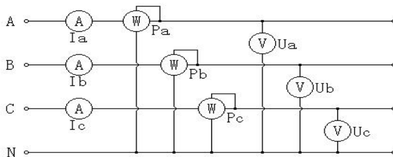
图二十、三相四线计量原理图
