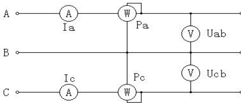
图十九、三相三线计量原理图
